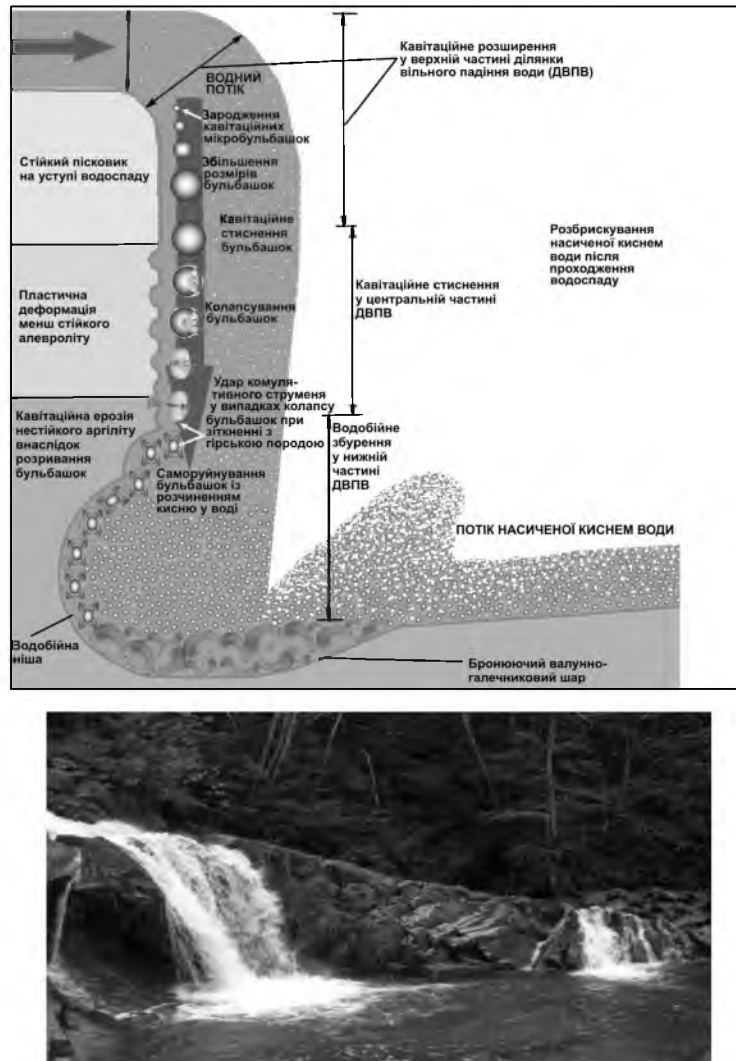
Рис. 1. Модель (вгорі) та водоспад на р. Кам'янка (внизу) як приклад гідродинамічного бар'єру з кавітаційним розширенням та стисненням, водобійним збуренням водного потоку на різних ділянках вільного падіння води, зародження кавітаційних бульбашок, збільшення їхніх розмірів та колапсування з ерозійним впливом при ударі кумулятивного струменя, насиченням води киснем при саморуїнуванні бульбашок, розбризкування та потоку води збагаченої розчиненим киснем
