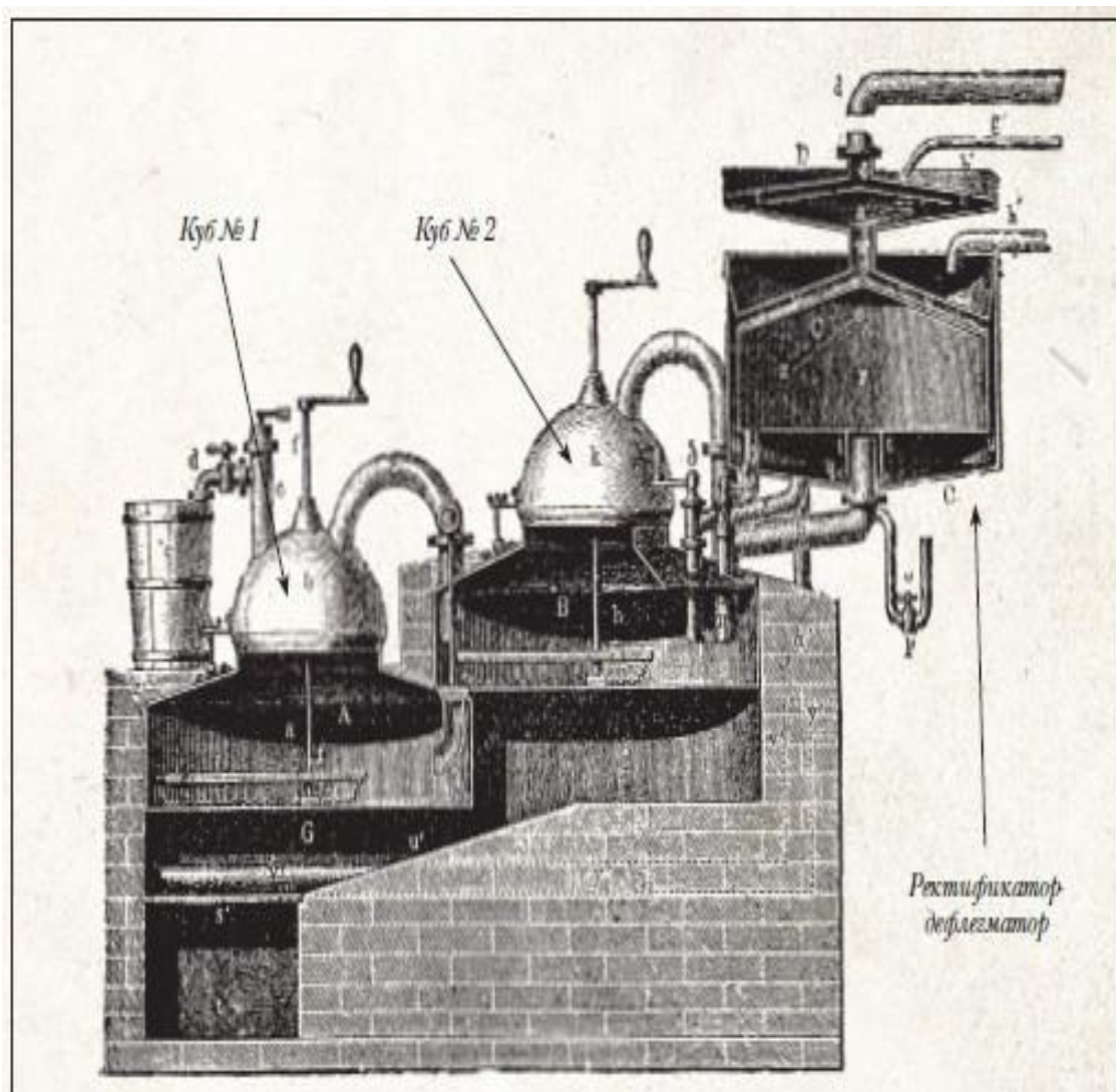
Аппарат Писториуса
